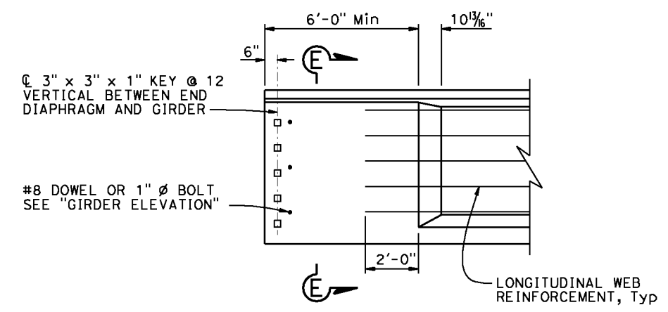
OPTIONAL END BLOCK - ELEVATION
