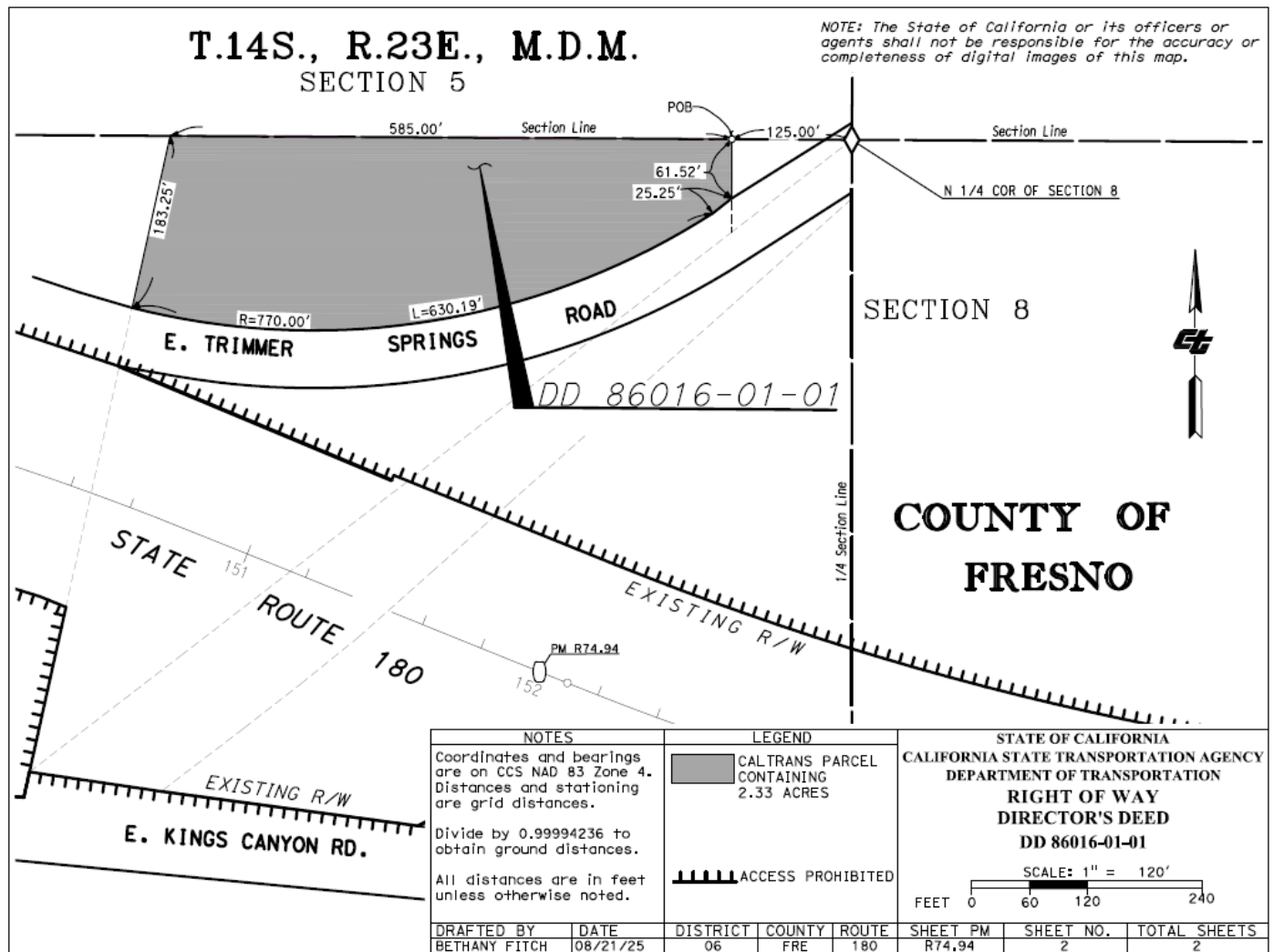
86016-01-01 Director's Deed Parcel Map
