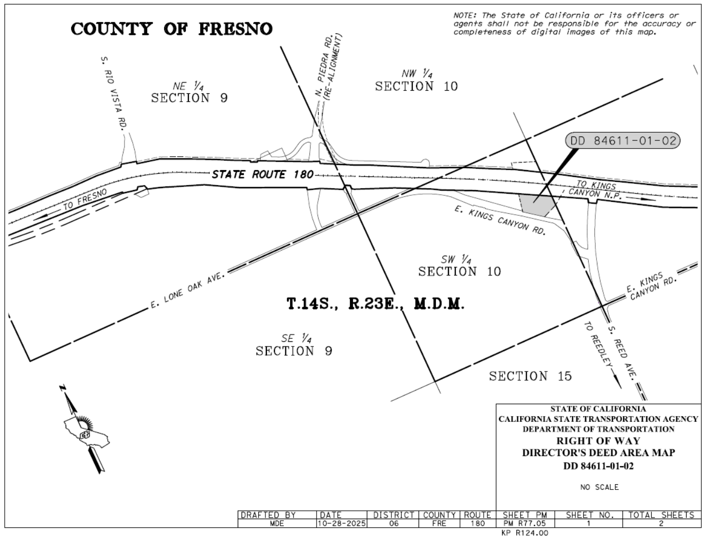
DD 84611-01-02 Parcel Map
