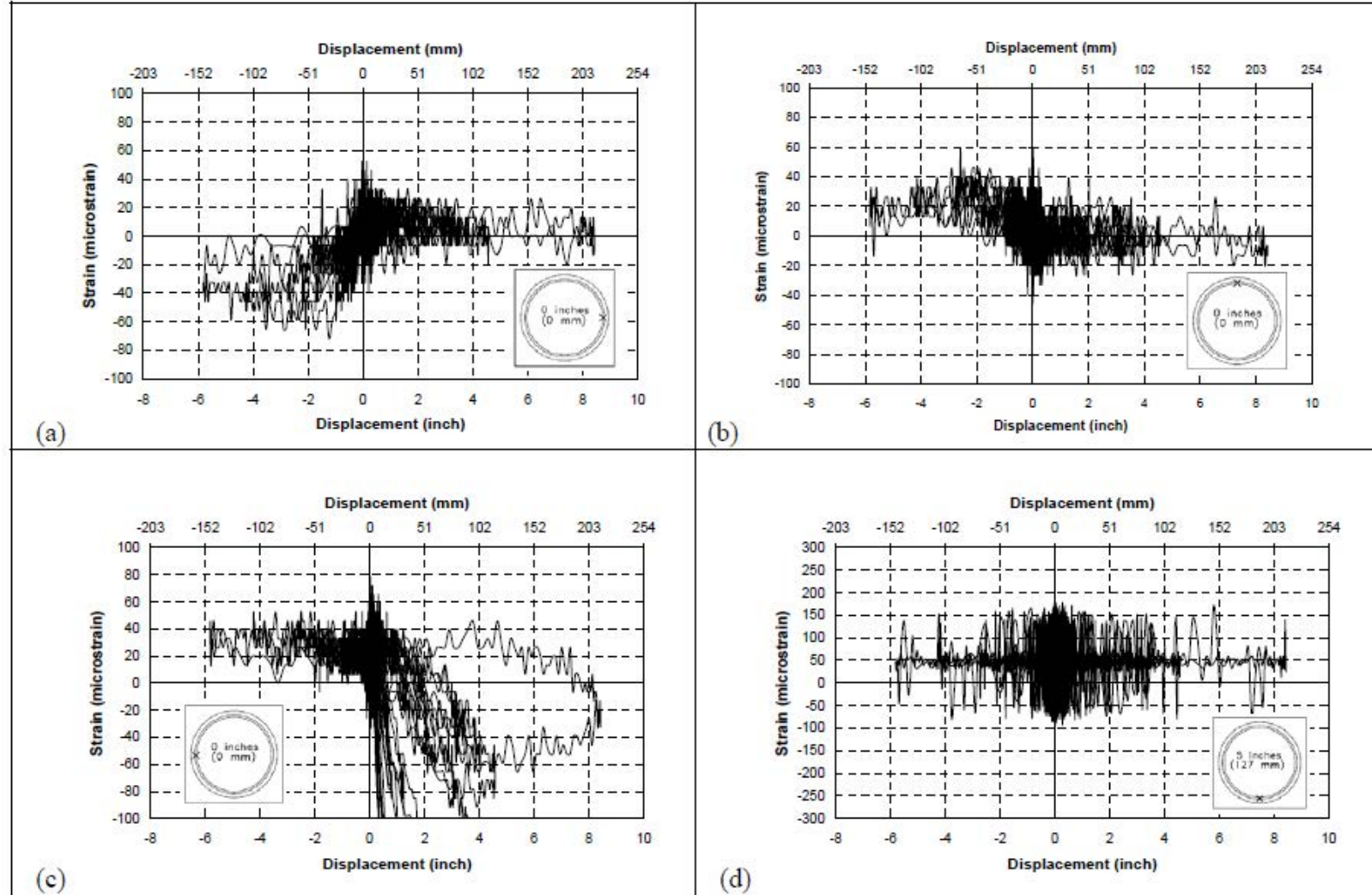
Fig. A-11. a) sg 44, b) sg 45, c) sg 46, d) sg 47 in SC-2
